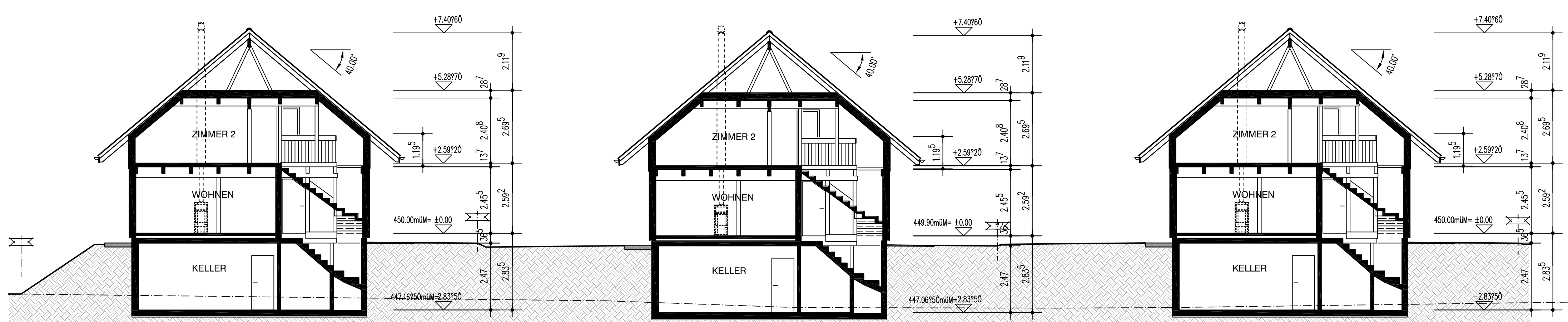
R4 QUERSCHNITT
